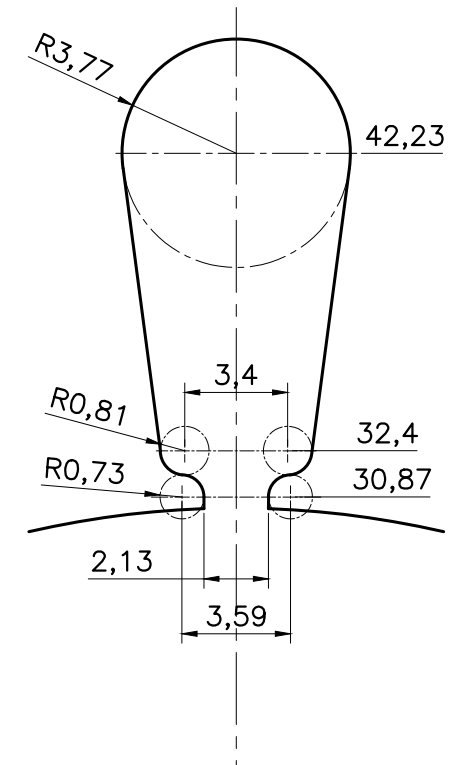
DETALLE DE LA RANURA B (20 ranuras) Escala 4:1
